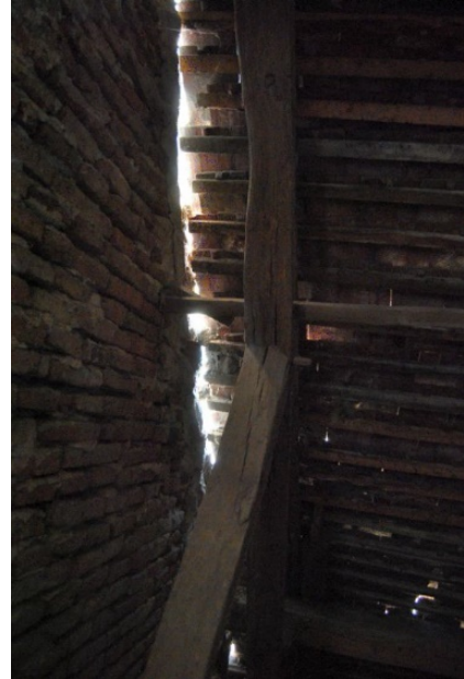
Abb. 38 – Langhaus, defekter Anschluss Dach-Turm
